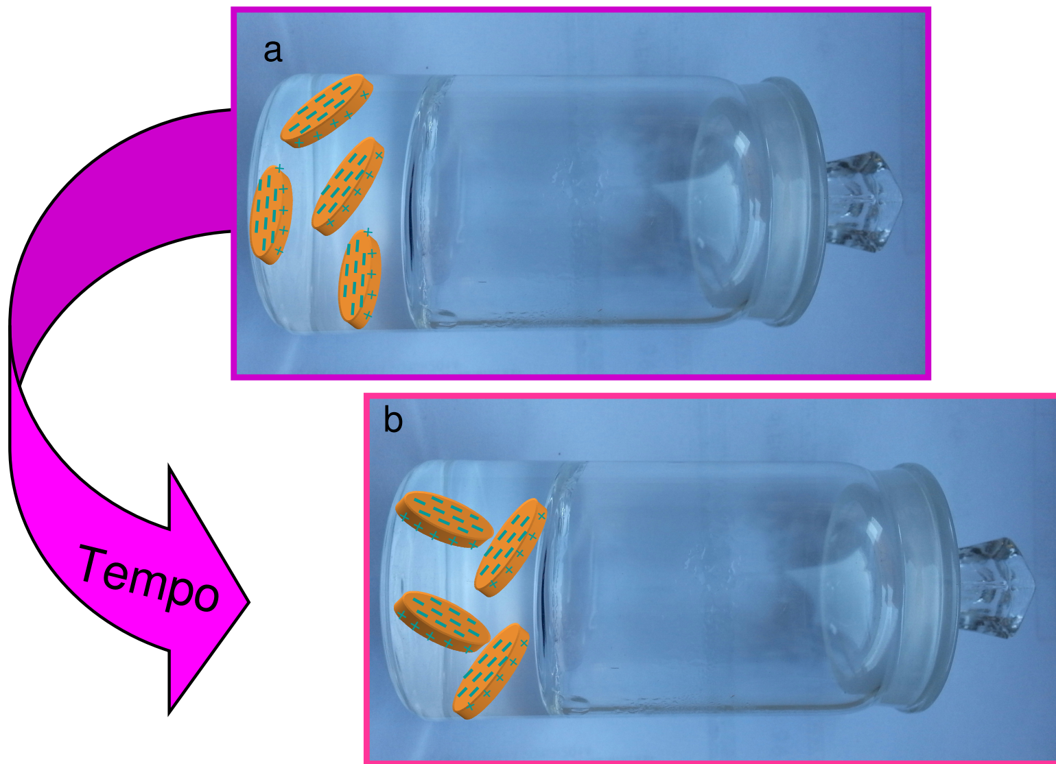
Fig: Rappresentazione schematica della trasformazione spontanea di un'argilla colloidale da un vetro costituito da particelle discoidali disordinate nelle posizioni e negli orientamenti (a) ad un nuovo vetro in cui i dischetti si orientano parzialmente a distanza a formare una struttura a 'castello di carte' (b).
